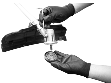
Fig. 10 – Montaje de la brida interna
