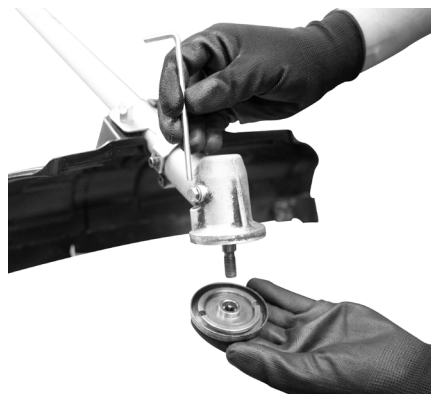
Fig. 6 – Montaje de la brida interna
